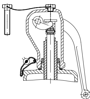
Test gag
