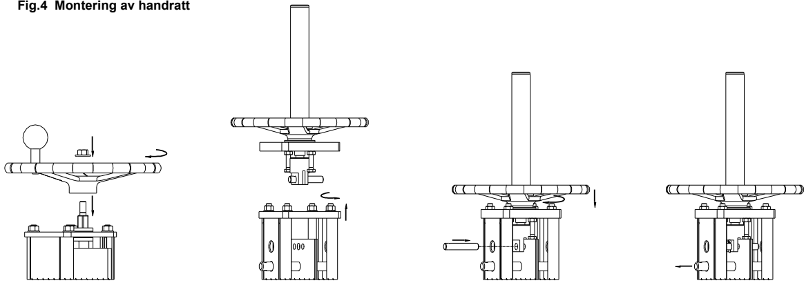
Fig.4 Montering av handrätt
